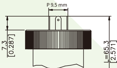
M-4 PIN 連接頭 EN 175301-803C
