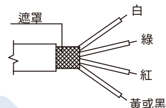
F-4 PIN 電纜
