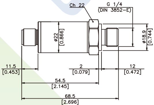
連接器 M12 × 1
