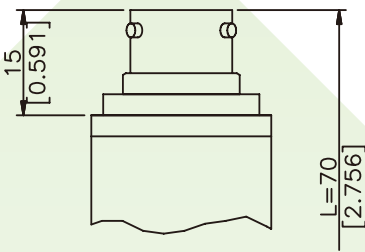
V-6 PIN 連接頭
