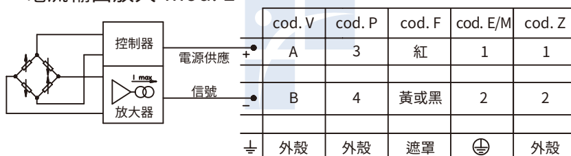
電流輸出放大-mod. E
